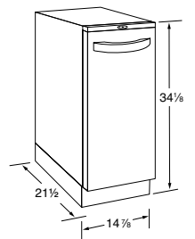
15XESS 15XEW
